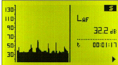
Schermata grafica in modalità di misura fonometro
